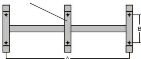
Maatvoering van de boorgaten van de ophangbeugel
